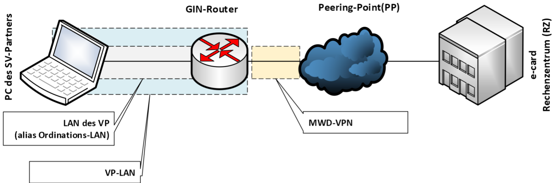
Abbildung 1: Schematische Darstellung vom GDA-LAN zum Rechenzentrum
